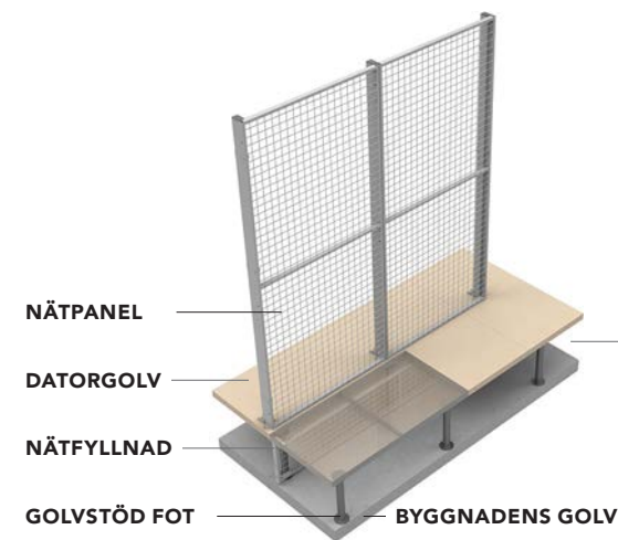
Ett exempel på utfyllnad mellan byggnadsgolvet och datorgolvet.
