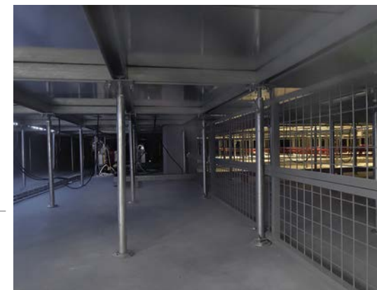
Ett exempel på utfyllnad mellan byggnadsgolvet och datorgolvet.
