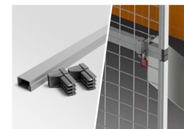
11 KAPNINGSPROFIL Detta är ett användarvänligt och flexibelt sätt att justera höjden på nätpaneler vid montering utan att systemet förlorar i styrka.
